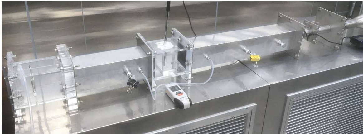
ガス除去フィルタ試験装置
